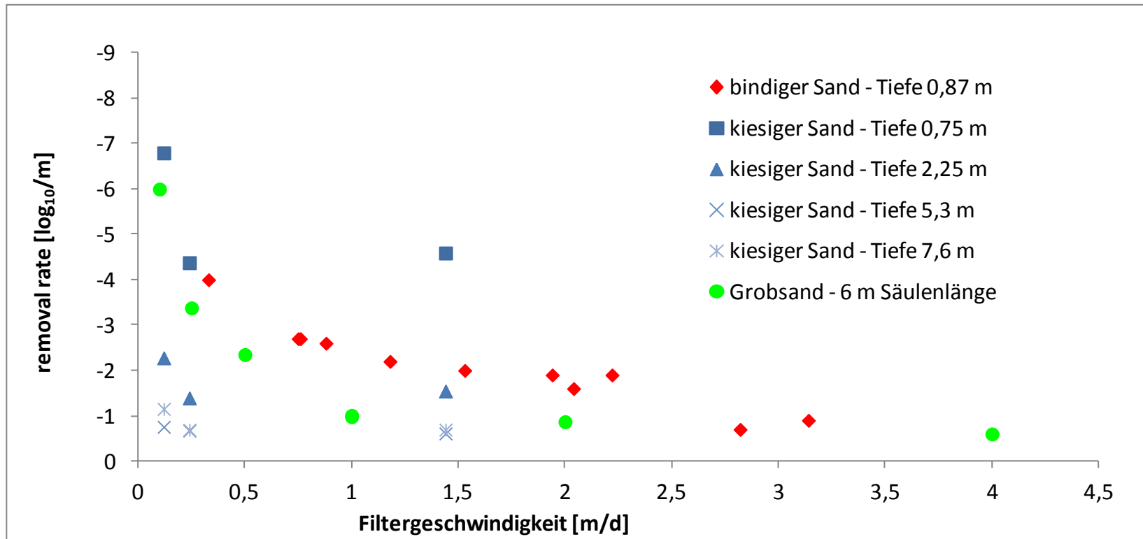
Abbildung 1: Removal rates in Abhängigkeit der Filtergeschwindigkeit (Vaughn et al., (1981; kiesiger Sand), Wang et al., (1981; bindiger Sand), Lopez et al., (in prep., Grobstand))
